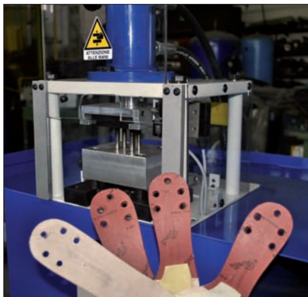
PARTICOLARE DEL DISPOSITIVO DI FORATURA
